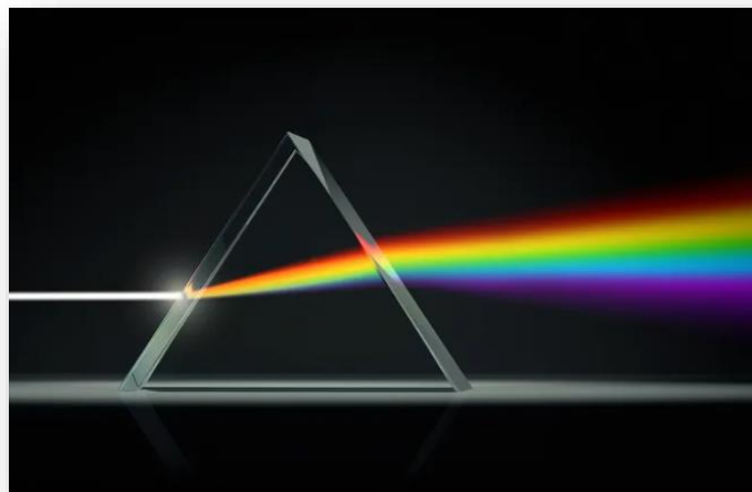
La diffraction d'un rayon de lumière à travers un prisme
