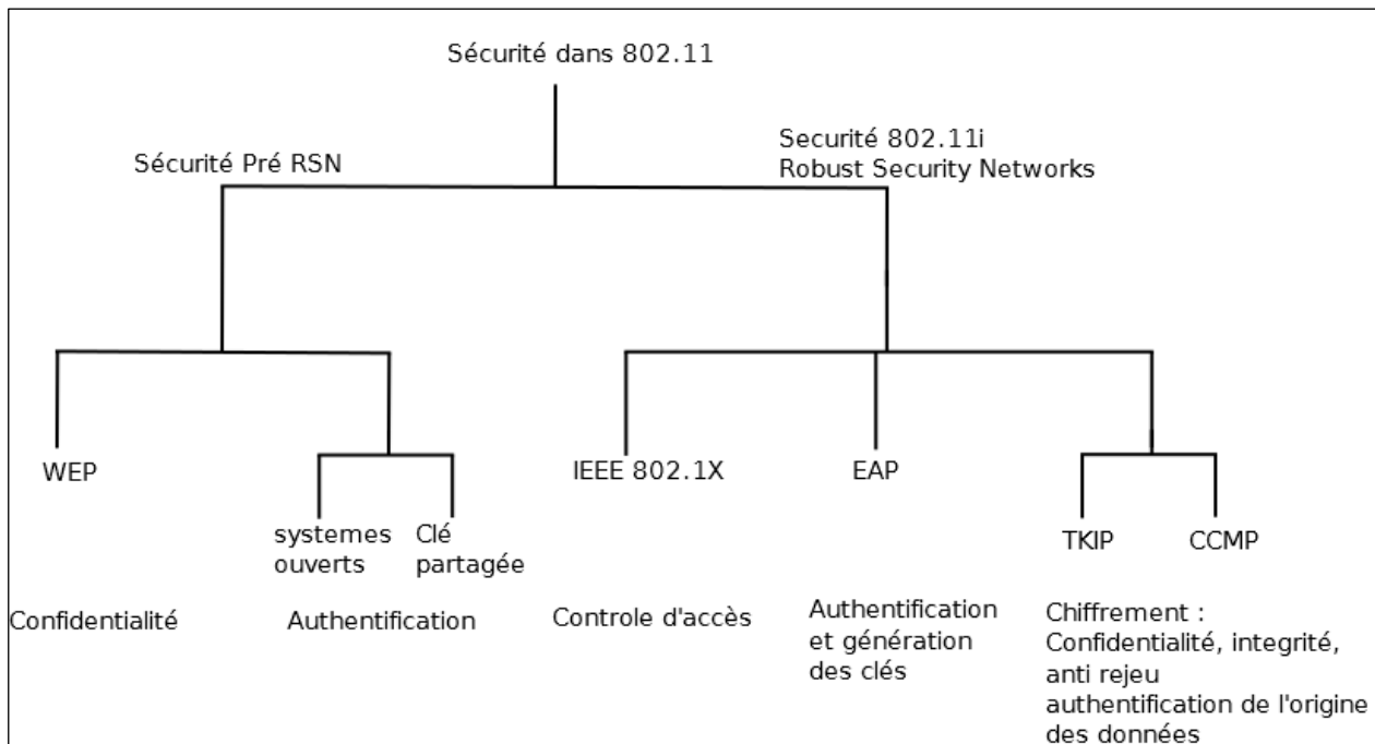
Figure 3 : Sécurité 802.11
